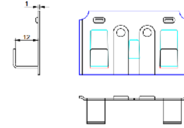
PASLANMAZ YATAY(ALT) İKİLİ KLİPS
