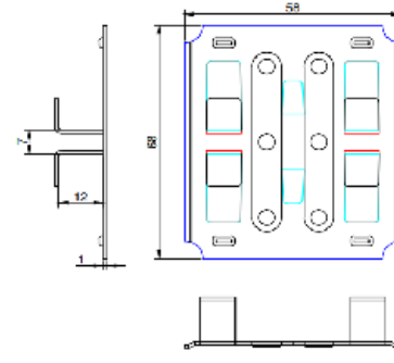
PASLANMAZ DÖRTLÜ KLİPS
