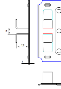
PASLANMAZ DİKEY İKİLİ KLİPS
